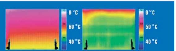
A Plan radiátor és egy másik, sík dekorlemezzel ellátott radiátor hőfényképe
